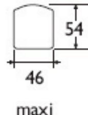
Mått på kabelanslutning i Botten.
